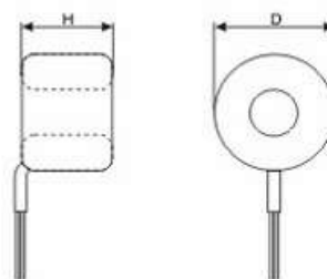
External Dimension 外形尺寸
