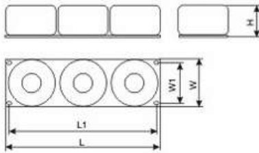
External Dimension 外形尺寸(A)
