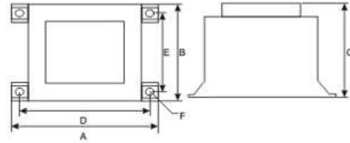
External Dimension 外形尺寸
