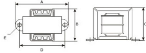
External Dimension 外形尺寸
