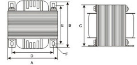
External Dimension 外形尺寸
